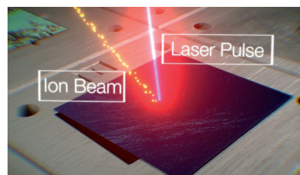
Obr. 2: Koincidentní FS laser a iontový paprsek MAGCIS.
