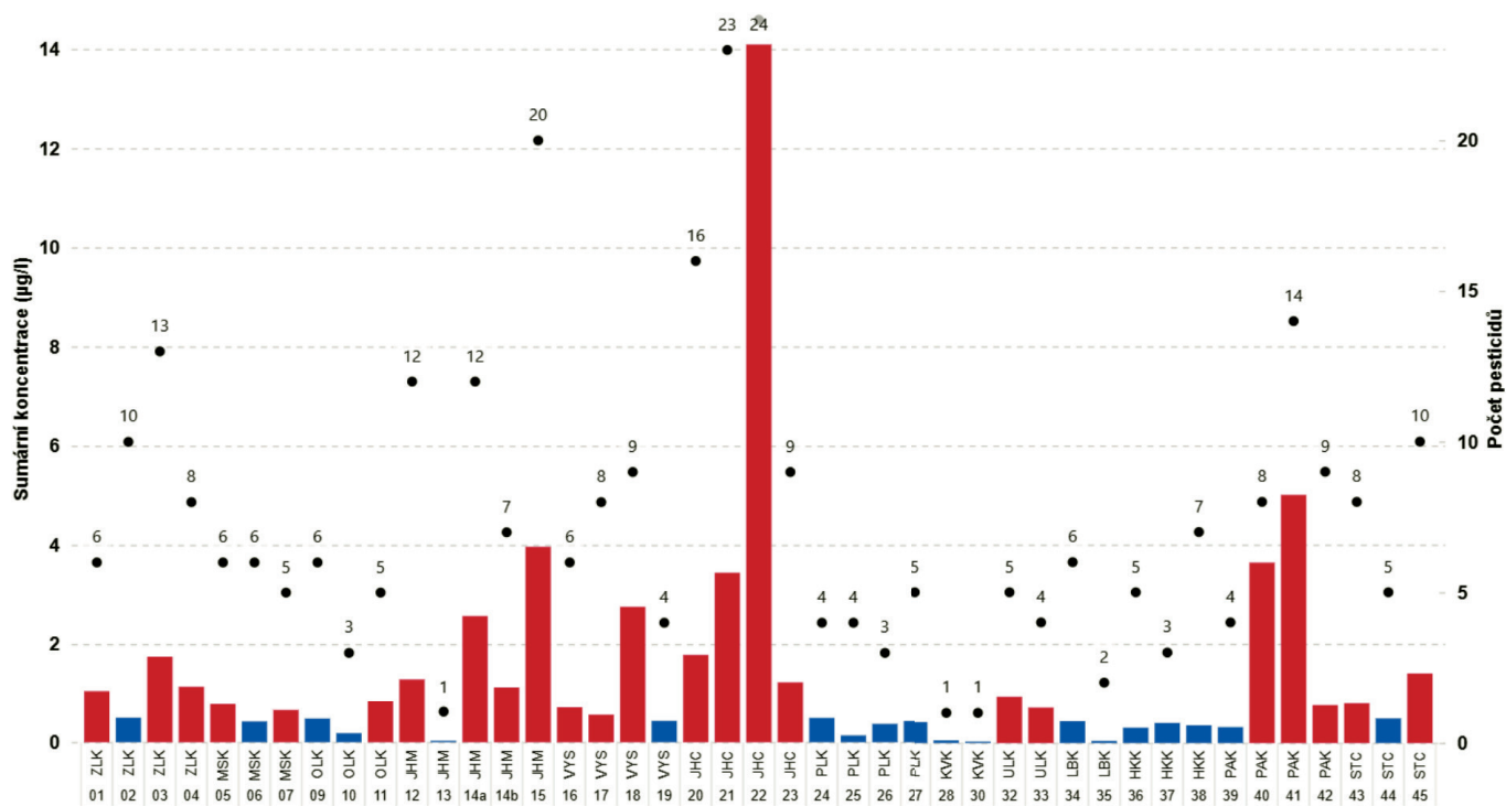
Obr. 2: Pesticidy v povrchových vodách České republiky (µg/l). Červeně jsou vyznačeny koncentrace, které nevyhověly limitní hodnotě.
